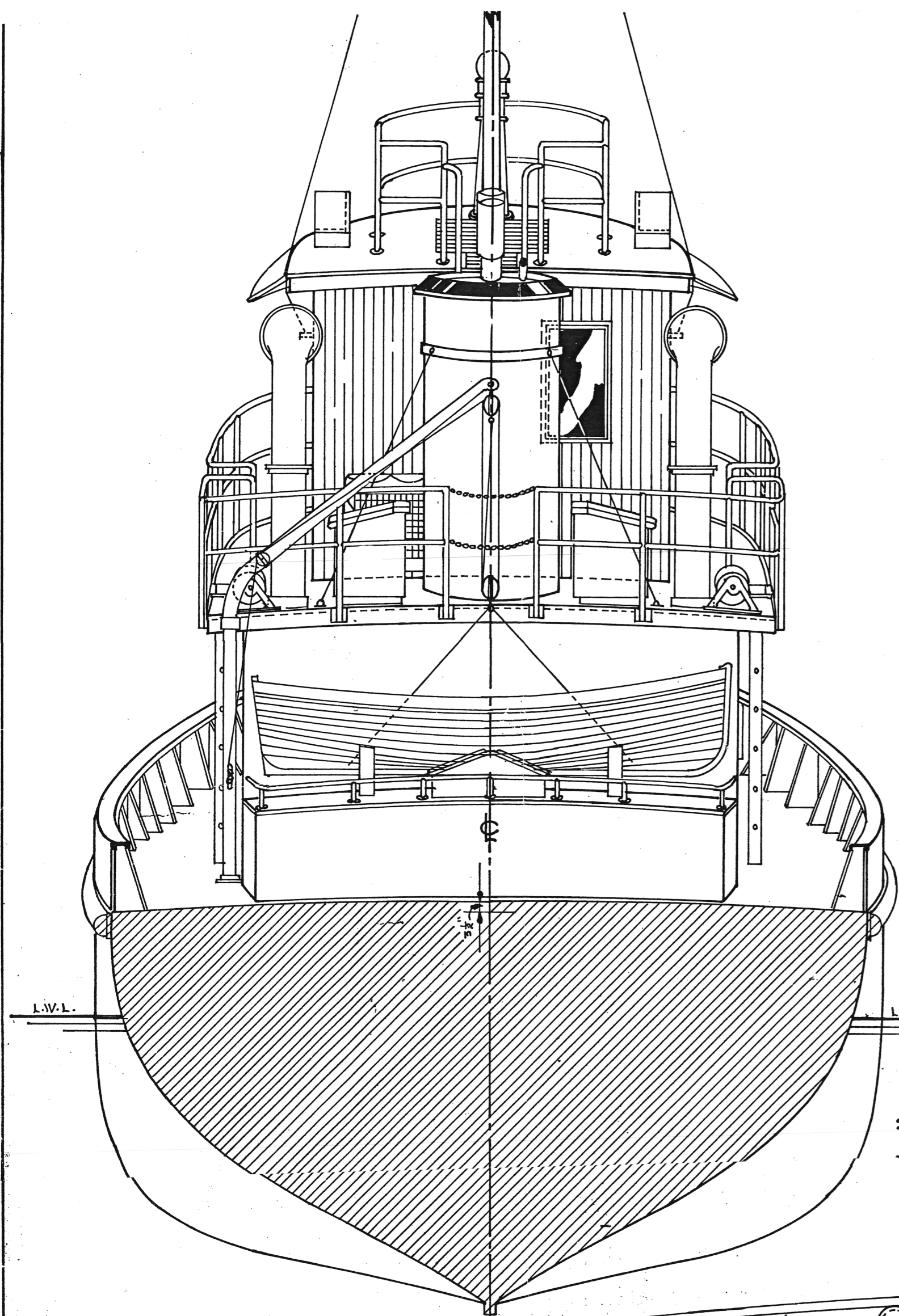
SECTION A-A
